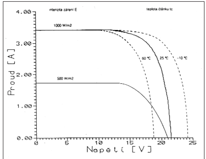
Obr.6 Charakteristika modulu M-S36-53
