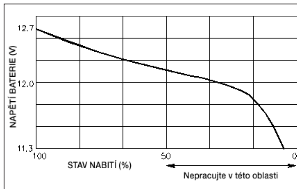
Obr.4 Napětí baterie versus stav nabití. Plně nabitý olověný akumulátor má napětí asi 12,7 V. Jak se baterie vybití, toto napětí klesá. V praxi je dobré udržovat staniční (deep-discharge) baterii nad 50% kapacity - tím se udrží napětí nad úroveň 12 V. Tato charakteristika se liší podle baterie a vzhledem k teplotě a velikosti vybíjení.
